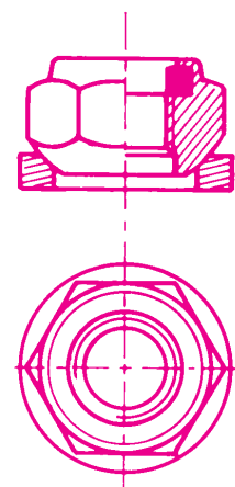
Porca de vão esférica autofreada ROTULAGEM \pm 8^\circ
