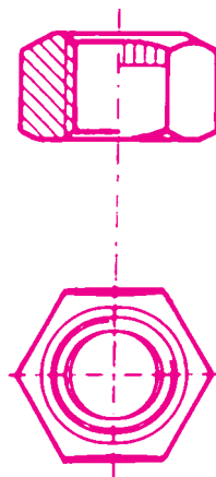
Porca cônica autofreada
