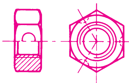
Porca sextavada autofreada (DIN 980)
