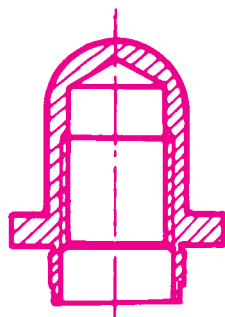
Porca cega de incrustar
