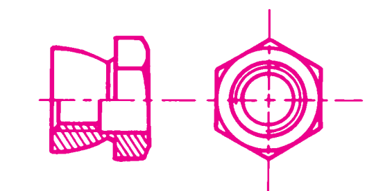
Porca inviolável autoquebrável
