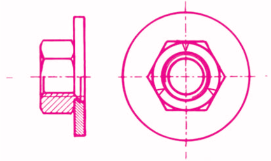
Porca autofreada com arruela plana móvel
