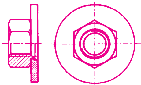
Ecrou à rondelle plate mobile
