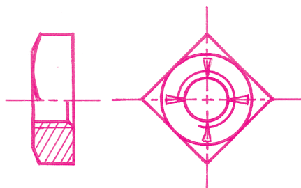
Ecrou carré auto-freiné
