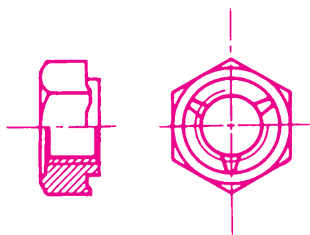
Ecrou à souder auto-freiné
