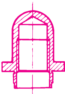
Ecrou borgne à sertir
