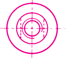
Canon taraudé auto-freiné
