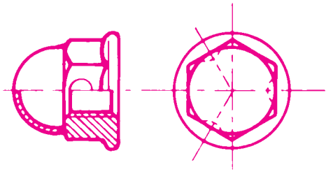
Ecrou borgne à embase auto-freiné
