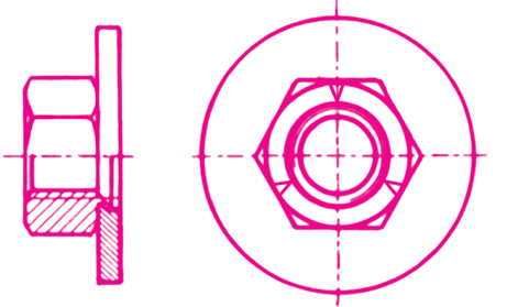
Ecrou auto-freiné à rondelle plate mobile
