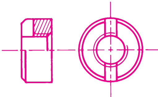
Ecrou rond à encoche
