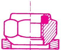
Ecrou à portée sphérique auto-freiné ROTULAGE \pm 8^\circ
